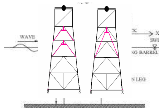
الف) کاربرد میراگر فلزی در سکوی جکت ب) کاربرد میراگر نوع TLD در سکوی شناور از نوع پایه
