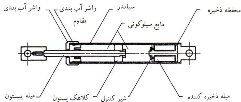
شکل ۱۰- ساختمان یک میراگر سیال لزج
