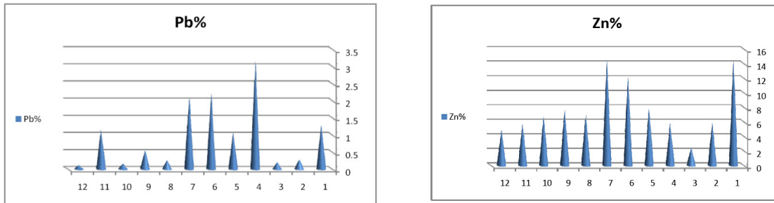
شکل ۵- چگونگی توزیع عناصر سرب و روی
