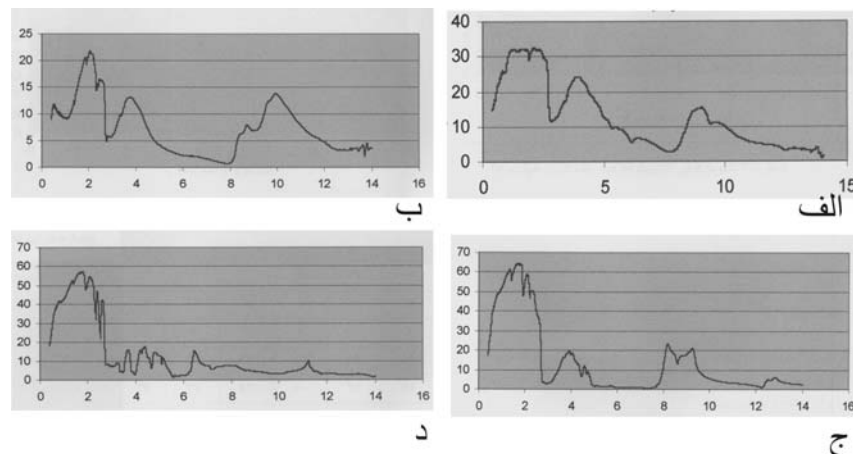
شکل ۳- نمودارهای طیفی که بر روی محور افقی طول موج بر حسب میکرومتر و بر روی محور قائم در صد انعکاس می باشد. الف) نمودار طیفی تراکیت، ب) نمودار طیفی دیوریت، ج) نمودار طیفی ماسه سنگ، د) نمودار طیفی سنگ آهک.
