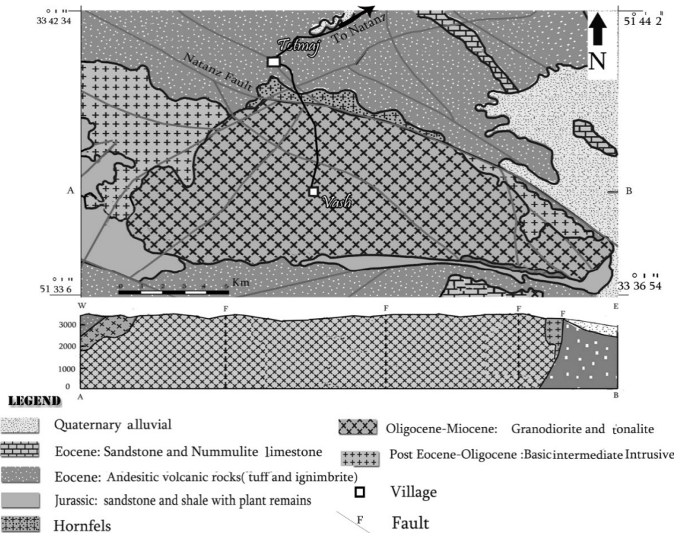
شکل (۱) نقشه زمین شناسی توده نفوذی وش با تغییرات از (عائلی مهابادی و همکاران ۱۳۷۷).
