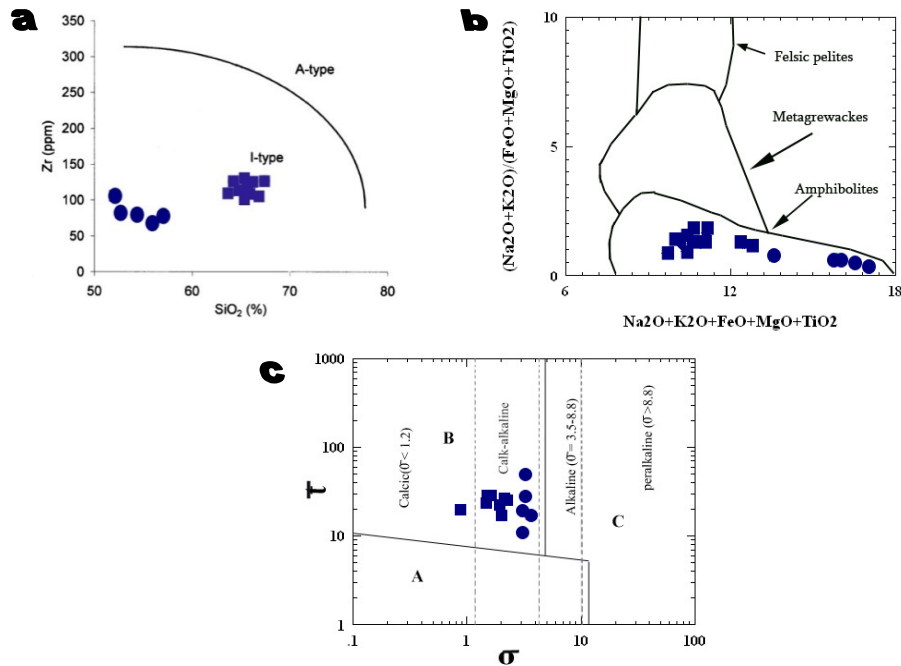
شکل ۴) a: نمودار متمایز کننده گرانیت‌های نوع I از گرانیت‌های نوع S بر حسب درصد وزنی \text{SiO}_2 به Zr b: نمودار تعیین نوع ماگما (\text{Na}_2\text{O}+\text{K}_2\text{O})/(\text{FeO}+\text{MgO}+\text{TiO}_2) در مقابل \text{Na}_2\text{O}+\text{K}_2\text{O}+\text{MgO}+\text{TiO}_2+\text{FeO} c: نمودار متمایز کننده نوع ماگما (گوتینی، ۱۹۸۶).
