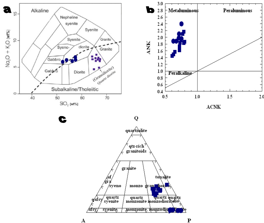
شکل 3) a: موقعیت قرارگیری نمونه های توده وش در دیاگرام QAP: طبقه بندی ژئوشیمیایی و نامگذاری سنگها با استفاده از نمودار مجموع آلکالی در مقابل سیلیس. C: موقعیت نمونه های توده نفوذی مورد مطالعه در دیاگرام A/CNK در مقابل A/NK.
