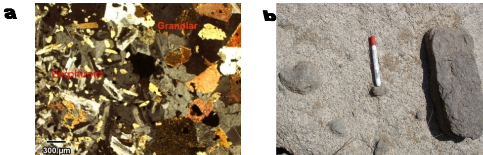
شکل (۲) a: دو بافتی بودن توده وش وجود بافت گرانولار و پورفیروئید در برونوم b: نمونه دستی برونوم با سنگ میزبان
