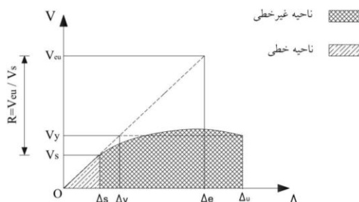
شکل (2): محدوده خطی و غیرخطی در منحنی ظرفیت سازه
