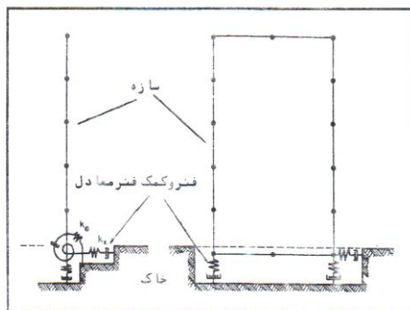
شکل 3 - مدل تحلیلی اندرکنش سازه - خاک با در نظر گرفتن انعطاف پذیری خاک به کمک فنرهای معادل
