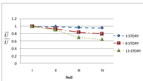
شکل 8 - نسبت ماکزیمم تغییر مکان نسبی طبقات در دو حالت تکیه گاه صلب و انعطاف پذیر.
