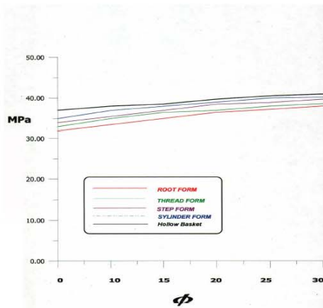
منحنی ۲: مقایسه ماکزیمم تنش در مدلها برحسب تغییر درجه
