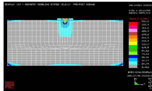
شکل ۲: مدل المان محدود
