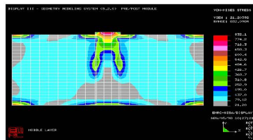
شکلهای ۳، ۴، ۵، ۶: توزیع تنش در مدلها
