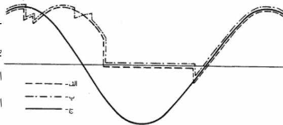
شکل (۱): ولتاژ پل اینورتر در حالت‌های الف) نقص آتش، ب) نقص کموتاسیون ناشی از کوچک بودن زاویه خاموشی و ج) بلوکه شدن اینورتر بدون مسیر کنارگذر [۶]
