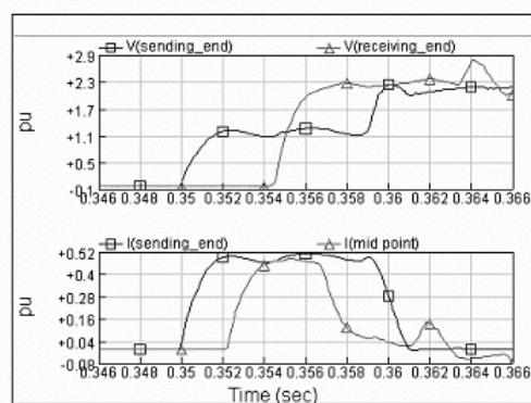
شکل (۱۴): شکل موج جریان ولتاژ در ابتدا، وسط و انتهای خط DC در شرایط راه اندازی با انتهای باز
