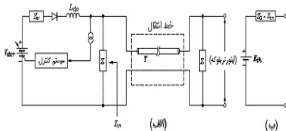
شکل (۳): الف) مدار معادل سیستم در زمان کلیدزنی خط DC ب) مدار معادل تونن ایستگاه مبدل از ابتدای خط DC
