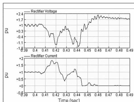
شکل (۱۲): جریان و ولتاژ طرف یکسوکننده پس از بلوکه شدن اینورتر (کنترل عادی)
