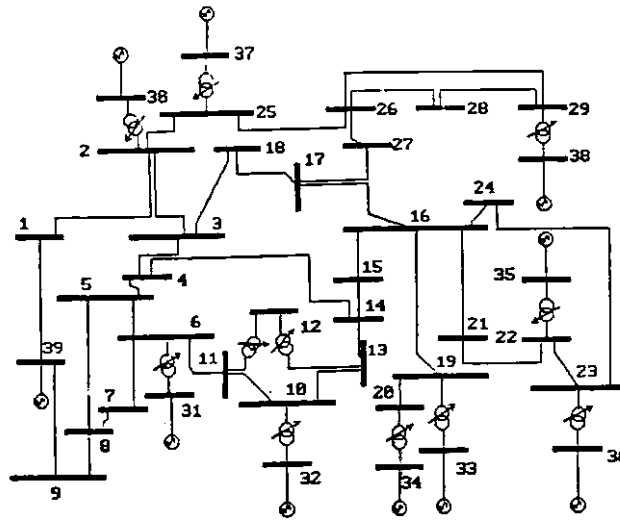
پیوست (۲): شبکه ۳۹ شینه IEEE
