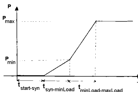
شکل (۱): مشخصه عمومی تولید توان واحدها
