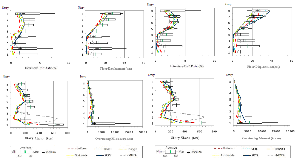
شکل (2): نتایج حاصل از تحلیل مدل هشت طبقه براساس روش های ضرائب FEMA-356 و طیف ظرفیت آیین نامه ATC-40
