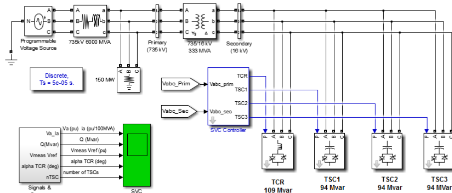
شکل ۴- مدار نمونه شبیه سازی SVC
