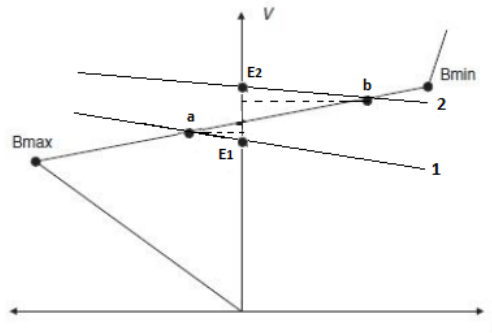
شکل ۲- پاسخ گذرای SVC
