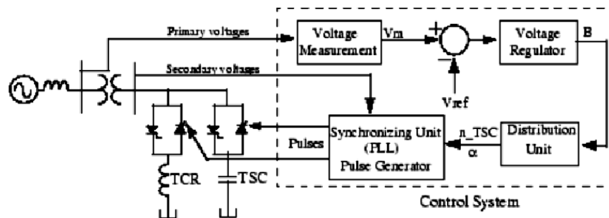
شکل ۳- دیاگرام تک خطی از یک نمونه SVC
