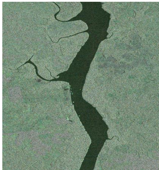
شکل ۲- تصاویر رنگی پائولی RGB ناحیه پانگ کالامبون در جنوب اندونزی
