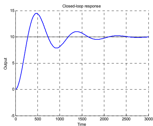
شکل ۱۴ پاسخ فشار درام P ( \text{kg/cm}^2 ) حول نقطه کار به ازای پارامترهای اولیه کنترل‌کننده
