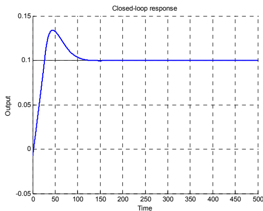
شکل ۹ پاسخ سطح درام (L (m)) حول نقطه کار به ازای پارامترهای اولیه کنترل کننده
