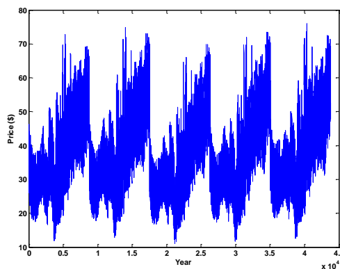
شکل ۹: قیمت ساعتی برق (پیش‌بینی شده در ۵ سال)
