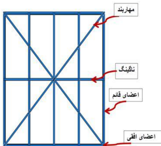
شکل ۴: معرفی اعضای قاب مهاربندی سرد نورد شده [۷]
