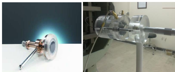
الف) نمایی از اتافک یونش ساخته شده با حجم متغیر ب) نمایی از اتافک یونش با حجم متغیر ساخت PTW
