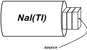
شکل ۴: هندسه آزمایش انجام شده
