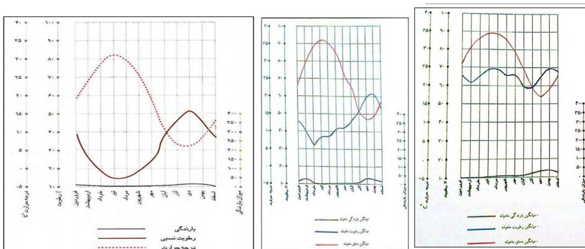
شکل (۳) میانگین دما، رطوبت و بارندگی در جیرفت (ملایی سربیزن، طیار، ۱۳۹۴)
