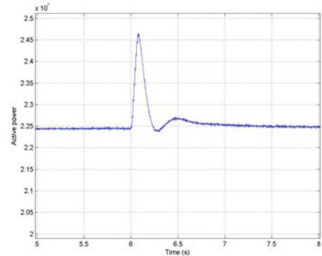
شکل (۷): توان حقیقی به ازای تغییر در ولتاژ مرجع
