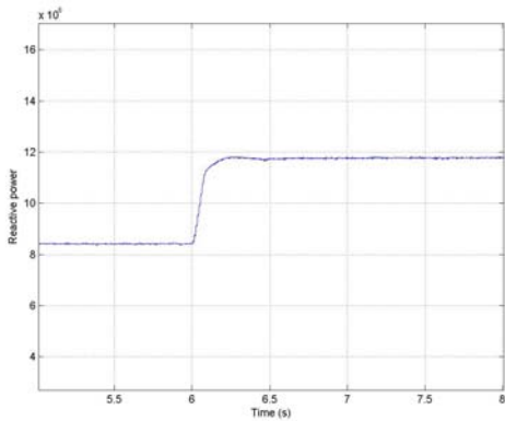
شکل (۸): توان موهمی به ازای تغییر در ولتاژ مرجع
