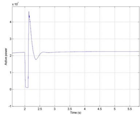
شکل (۳): توان حقیقی به ازای خطای اتصال کوتاه
