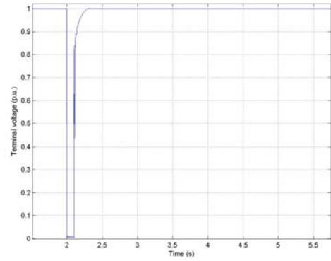
شکل (۱): ولتاژ ترمینال به ازای حالت اتصال کوتاه
