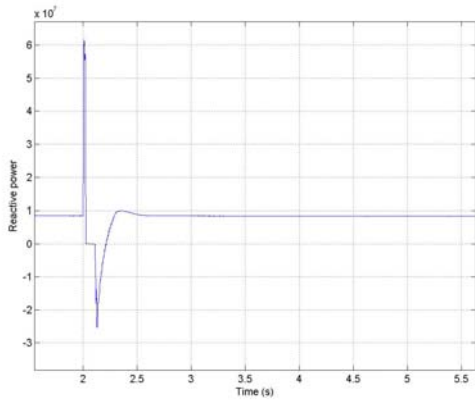
شکل (۴): توان موهمی به ازای خطای اتصال کوتاه
