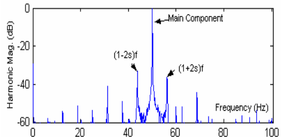
شکل ۷ طیف های فرکانسی جریان موتور جدید در حالت بارداری تا هارمونیک ۲۰ (بالا) و در اطراف هارمونیک ۵۰ هرتز (پائین)
