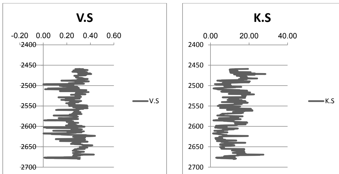
شکل ۶- نسبت پواسون
