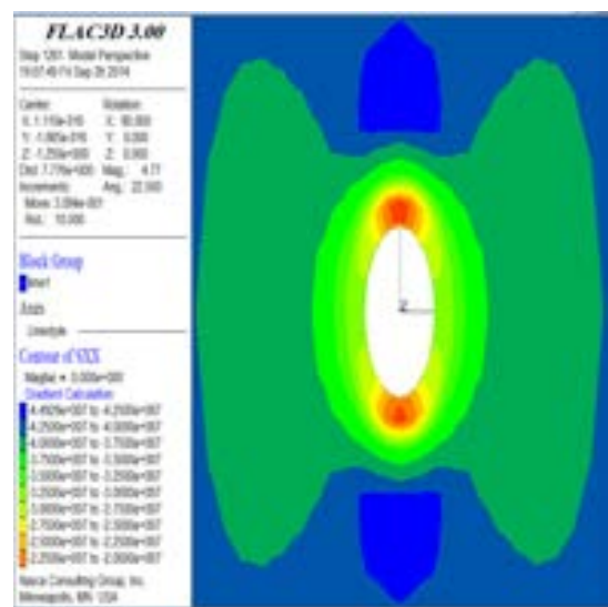
شکل ۳۰- توزیع تنش القایی حداقل در فشار گل (30 mpa)
