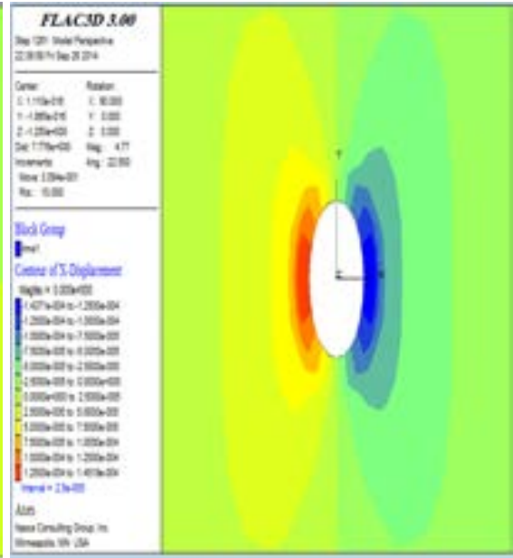
شکل ۲۸- جابجایی در جهت X در فشار (30 mpa)
