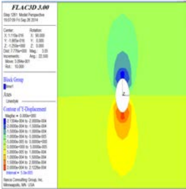
شکل ۲۹- جابجایی در جهت Y در فشار (30 mpa)
