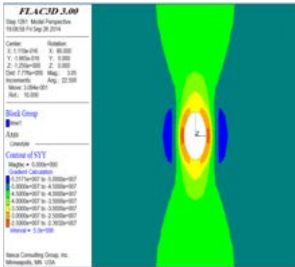
شکل ۳۱- توزیع تنش القایی حداکثر در فشار گل (30 mpa)
